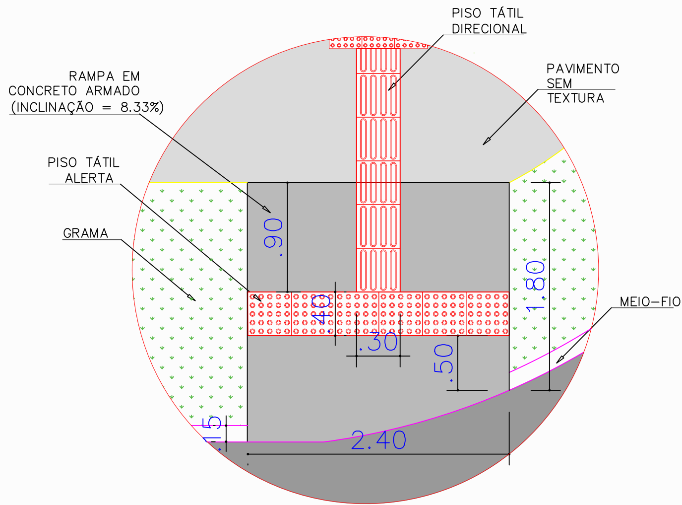
2 DET. 01 - RAMPA EM CURVA ESCALA 1:50
